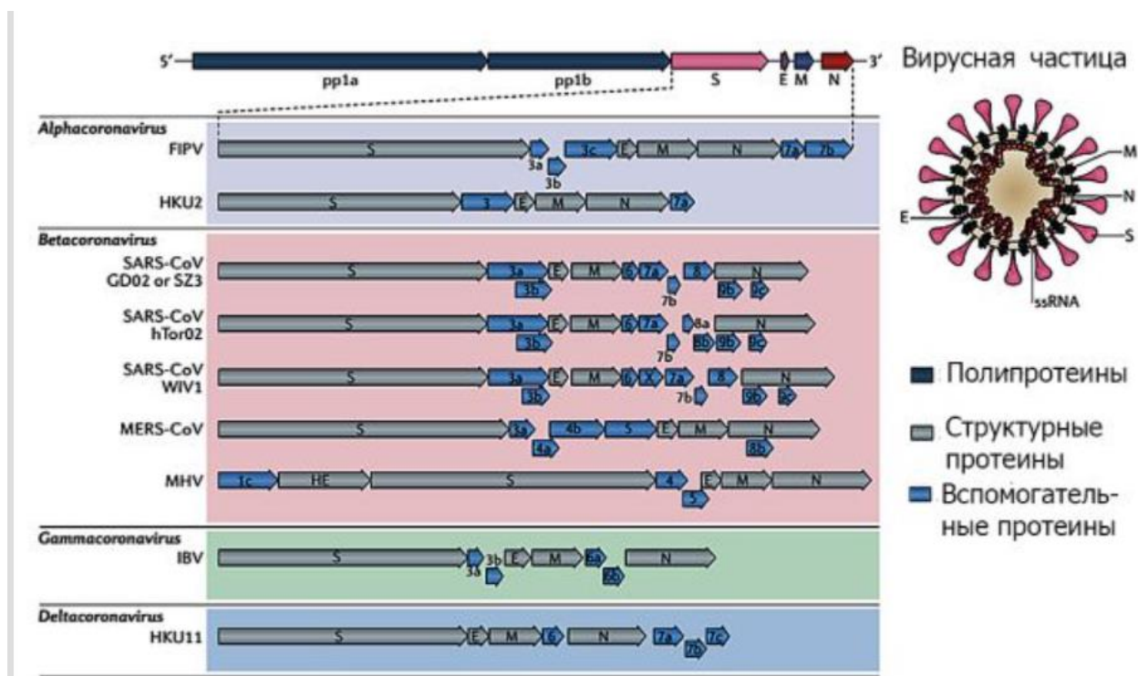
Рис.1 – Геномы коронавирусов типовых видов различных родов (по: М.В. Супотницкий, 2020 [1])
