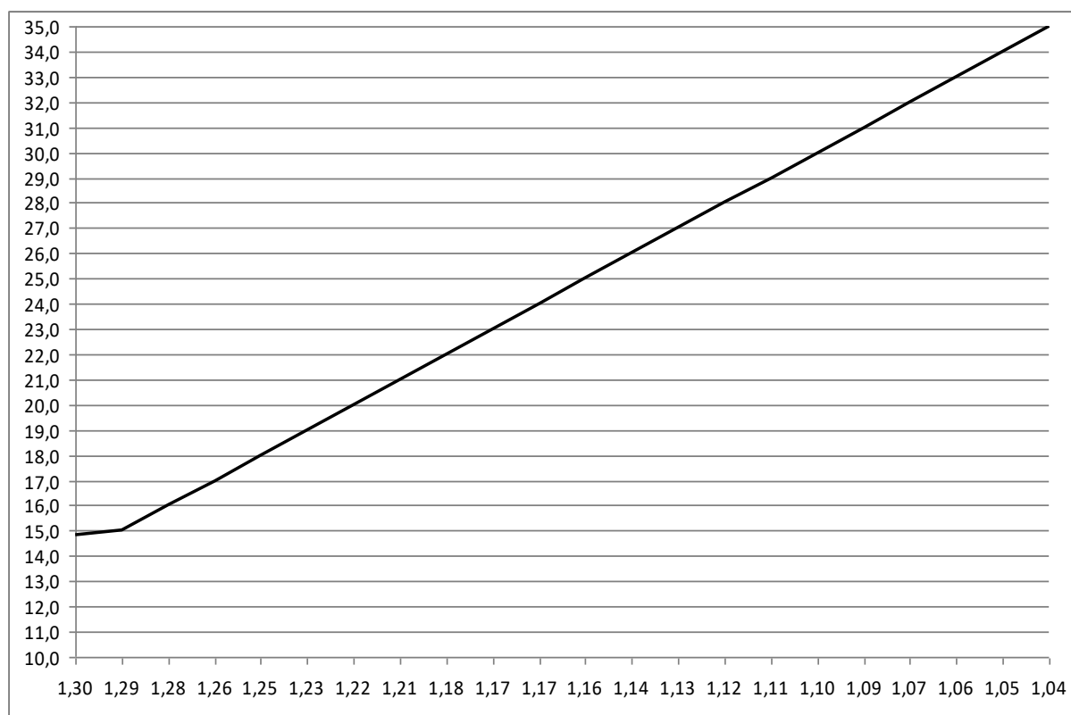
Рисунок 1 - «Зависимость» между влажностью и плотностью чернозема обыкновенного карбонатного (образец № 5)
